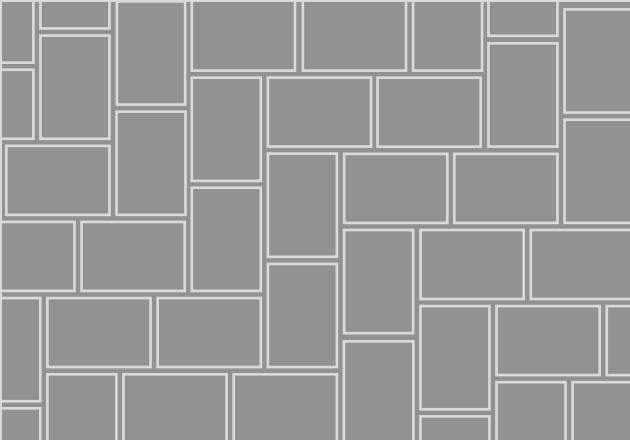
VERLEGEMUSTER FISCHGRÄTVERBAND
