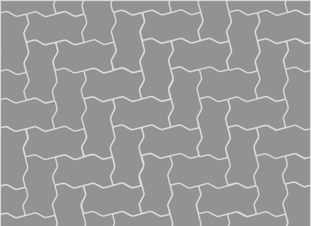
VERLEGEMUSTER FISCHGRÄTVERBAND ca. 125 x 93 x 8/10 cm // Microfase // 40 Normal- und 8 Halbsteine/Lage (Universal Fischgrät)
